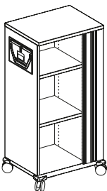
Höhe 1148 (3 OH), Breite 550, Tiefe 436 mm
