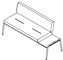
DOUBLE BENCH MIT ABLAGE SEITLICH | WITH SIDE TRAY 1.675 x 655 x 783 mm
