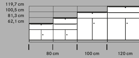
WINEA MAXX Regale mit versetzter Mittelseite WINEA MAXX bookcases with asymmetric separation panel
