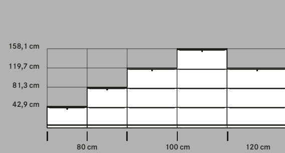
Hängehefterschränke, 1-3 Ordnerhöhen Hanging file cabinets, 1-3 file heights
