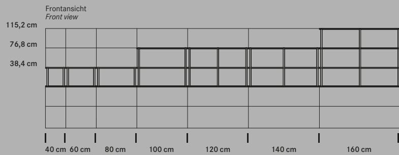
WINEA MAXX offene Aufsatzregale WINEA MAXX open top shelves
