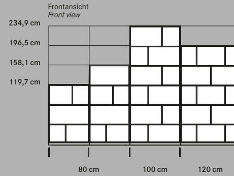
Flügeltüraufsätze, 1-4 Ordnerhöhen Upper double door cabinet parts, 1-4 file heights
