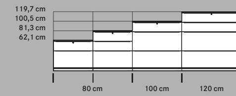
Regalaufsätze, 1-4 Ordnerhöhen Top racks, 1-4 file heights
