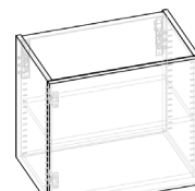
Oberschrank 525 / 1-Türig KKO6052T Höhe: 525 mm Breite(n): 350-600 mm mit 23 mm Griffüberschlag
