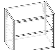
Oberschrank 525 / Regal KKO6052O Höhe: 525 mm Breite(n): 350-900 mm Tiefe: 380 mm
