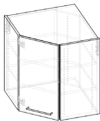
Oberschrank Eckschrank KKO6575E Höhe(n): 525 / 750 mm Breite: 650 / 650 mm mit Griff 224
