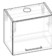
Oberschrank 525 / Lüfterbaustein KKO6052L Höhe: 525 mm Breite: 600 mm mit Griff 224
