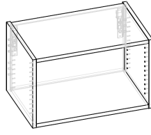
Oberschrank 375 / Regal KKO6037O Höhe: 375 mm Breite(n): 350-900 mm Tiefe: 380 mm
