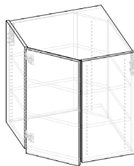
Oberschrank Eckschrank KKO6575E Höhe(n): 525 / 750 mm Breite: 650 / 650 mm mit 23 mm Griffüberschlag
