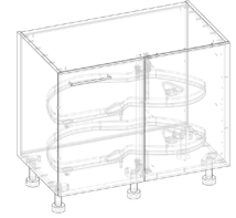
Unterschrank / LeMans KKU5090ELM Höhe: 725 mm Breite: 1000 mm
