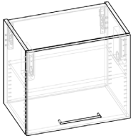
Oberschrank 525 / Klappe KKO6052K Höhe: 525 mm Breite(n): 350-900 mm mit Griff 224
