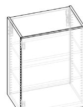
Oberschrank 750 / 1-Türig KKO6075T Höhe: 750 mm Breite(n): 350-600 mm mit 23 mm Griffüberschlag
