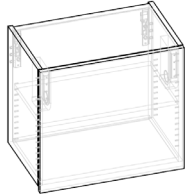
Oberschrank 525 / Klappe KKO6052K Höhe: 525 mm Breite(n): 350-900 mm mit 23 mm Griffüberschlag
