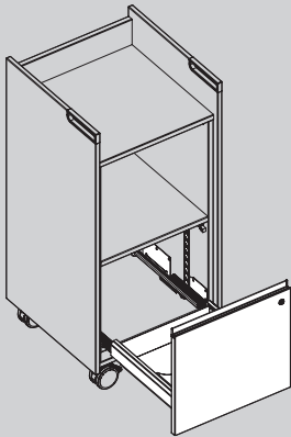
INNENLICHTEN 1 Lade
